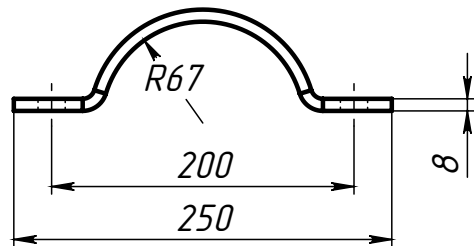
Поз.3 (Хомут)
