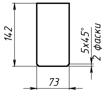
Поз.2 (Ребро)
